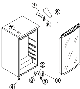
FIGURA 1 PORTA A ABRIR PARA A DIREITA
