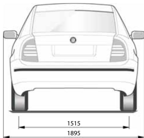
OBR. 8 ŠKODA SUPERB V ZÁKLADNÍCH ROZMĚRECH
