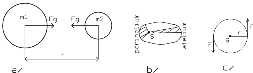
Obr 1.4 a) gravitační síla, b) 2. Keplerův zákon, c) dvojice síl
