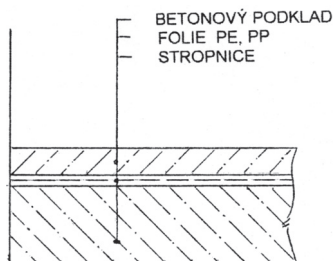
6 / Podkladní beton připojený na stropnicích
