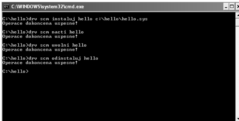
Obrázek 3.7: Použití drv.exe k manipulaci s ovladačem hello.sys
