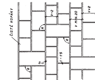
LÍC SVISLE PROVÁZOVANÉHO ČISTÉHO ZDIVA RÁDKOVÉHO.
