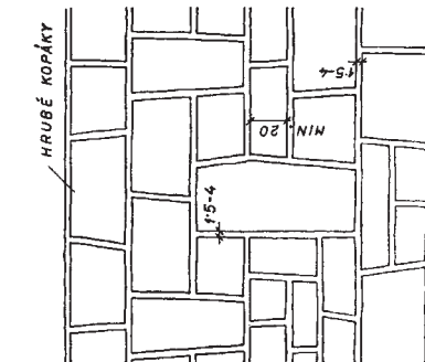
LÍC SVISLE PROVÁZOVANÉHO HRUBÉHO ZDIVA RÁDKOVÉHO.
