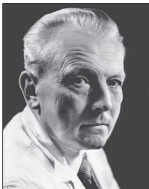
Obr. 1.2 Otakar Hněvkovský (1901–1980)
