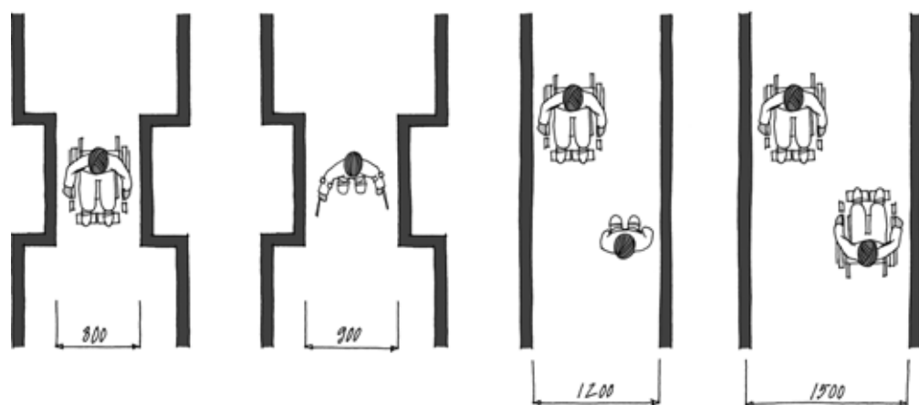
Obr. 1.4 Prostorové požadavky – chodby, průchody
