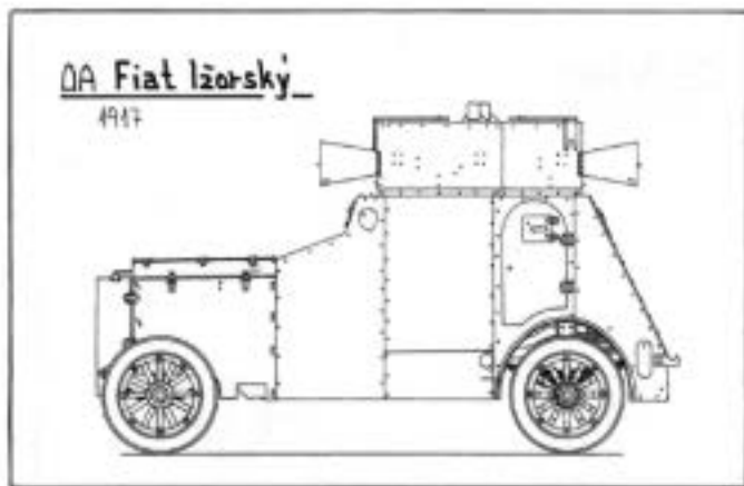
Ruský obrněný automobil Fiat, opancéřovaný v Ižorském závodě (nákres J. Suchý)
