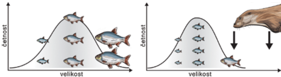
Obr. 2.3: Nasměřovaná selektce.
