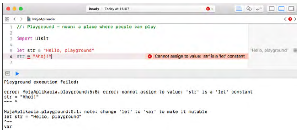
Obrázek 2.7: Pokus o přiřazení hodnoty do konstanty
