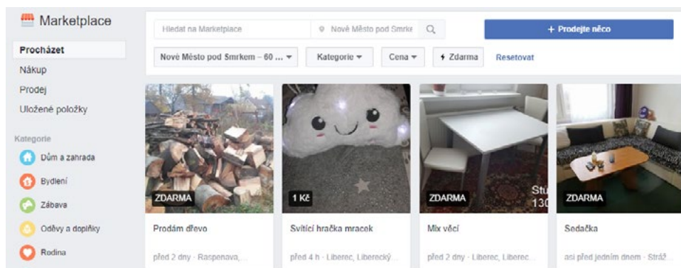
OBRÁZEK 2. 6. Marketplace
