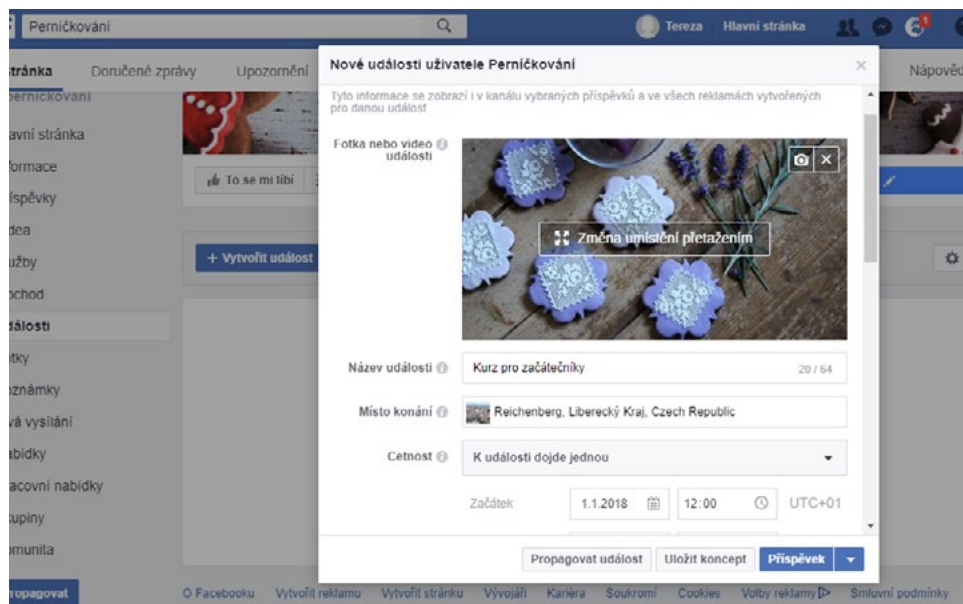
OBRÁZEK 2. 2. Vytvoření události
