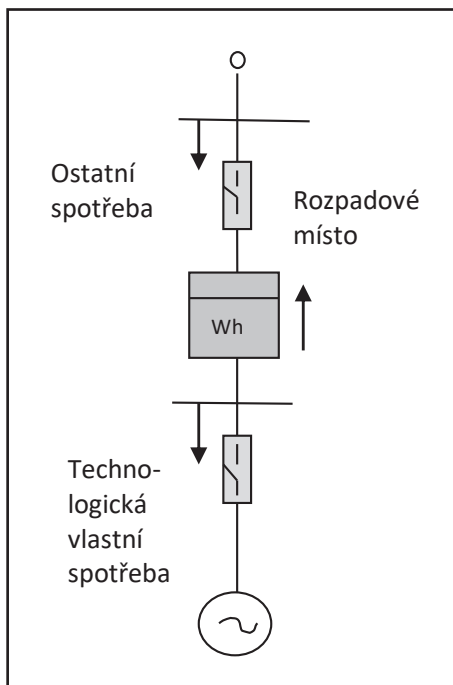
Obr. 2 Zapojení výroby (mikrozdroje) bez možnosti ostrovního provozu
