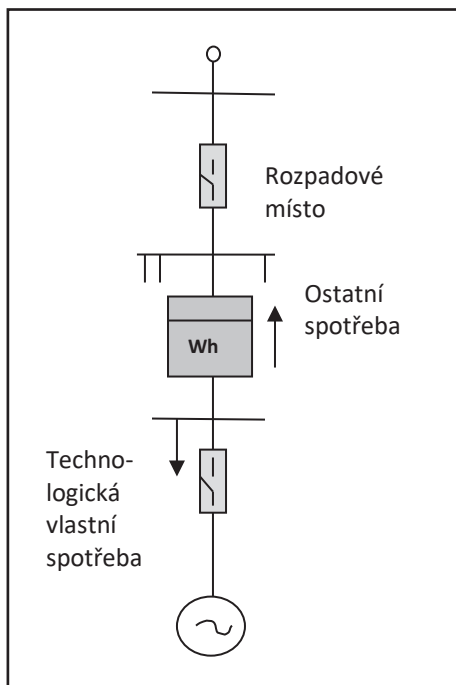
Obr. 1 Zapojení výroby (mikrozdroje) s možností ostrovního provozu
