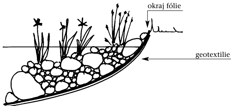
Obr. 8 K zakrytí okraje lze použít i geotextilii
