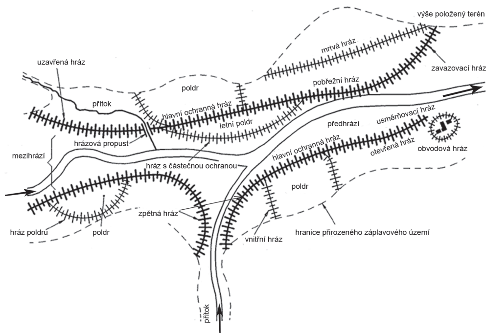
Obr. 1.1 Typy ochranných hrází (upraveno dle DIN 19712)
