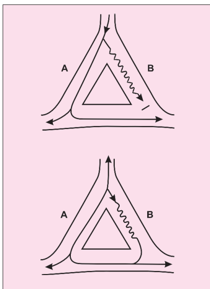
Obr. 3. Mechanismus vzniku arytmií - reentry mechanismus.
