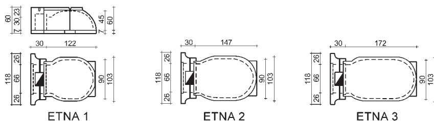
Obr. 9 Půdorys dna podlouhlého topného prostoru pece na pizzu typ Etna fy Edil Kamin
