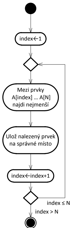
Obrázek 1.2: Diagram aktivit popisující první verzi algoritmu pro třídění pole
