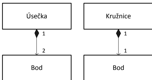
Obrázek 1.5: Znázornění vztahu mezi třídami Bod, Úsečka a Kružnice – čísla připojená ke spojnicím vyjadřují, že Kružnice obsahuje jeden Bod, zatímco Úsečka obsahuje dva Body
