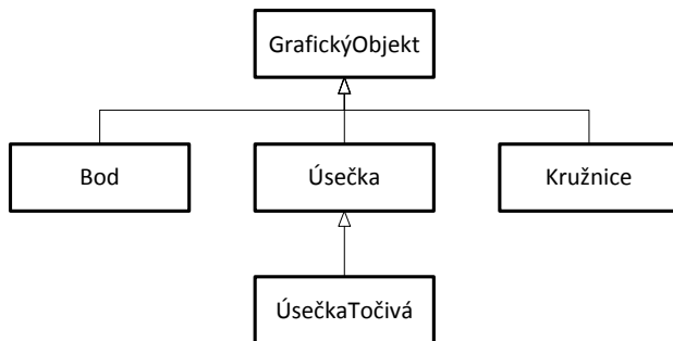
Obrázek 1.6: Dědičná hierarchie tříd z příkladu o grafickém editoru
