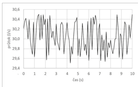
Obr. 4.1 Příklad záznamu „ustáleného“ průtoku čerpadlem
