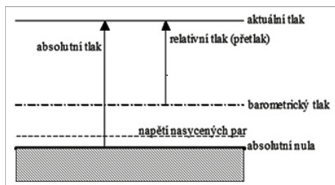
Obr. 1.2 Absolutní a relativní tlak
