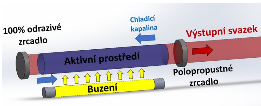
Obr. 1.1: Schematické znázornění základních prvků laseru
