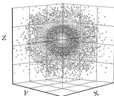
Obrázok 2. Elektrónový oblak atómu vodíka: časť trojrozmerného priestoru okolo atómového jadra, kde sa zachováva najväčšia pravdepodobnosť výskytu elektrónu.
