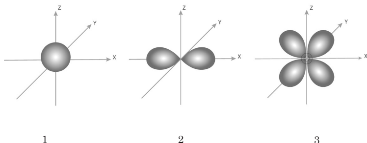
Obrázok 3. Rozličné formy elektrónového oblaku („geometria“ kvantovej chémie).
