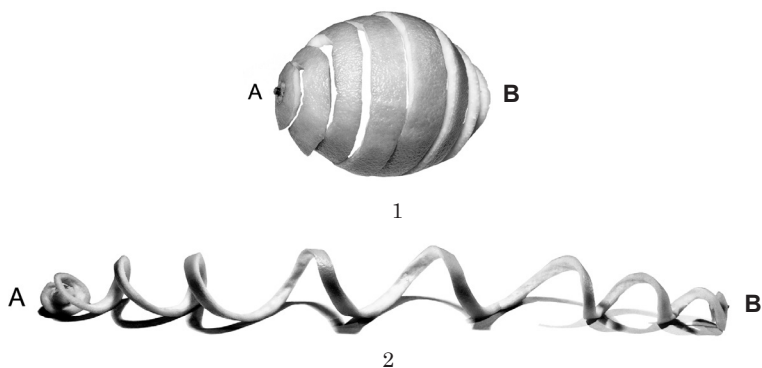
Obrázok 4. Názorný príklad premeny elektrónu z častice na vlnu:
