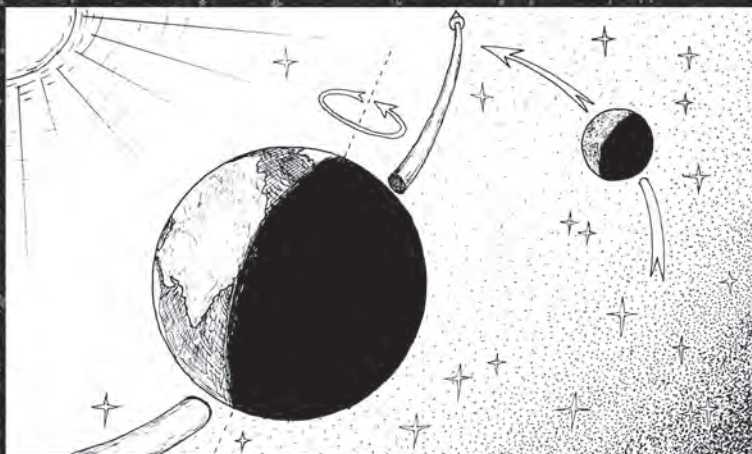
Tři základní astronomické oběžné doby, – den, měsíc a rok
