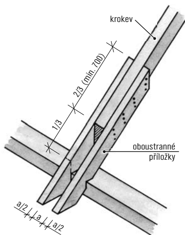
Obr. 10 Oprava uhnílého spodního konce krokve pomocí přílozek
