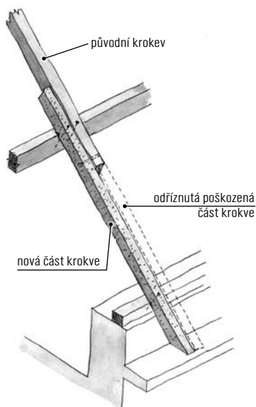
Obr. 7 Oprava krokve poškozené mezi pozednicí a vaznicí
