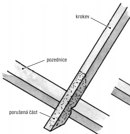
Obr. 9 Oprava uhnílého spodního konce krokev
