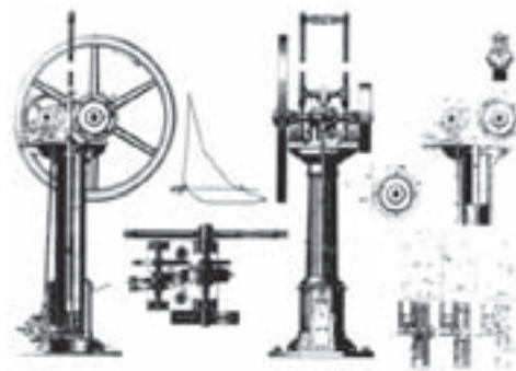
▲ Obr. 2.5 Plynový motor Nikolause Otta
