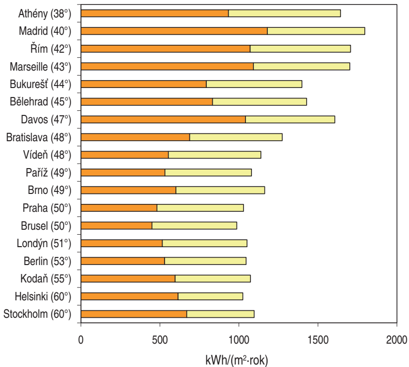
Obr. 1.7 Podíl přímého (tmavá) a difuzního (světlá) slunečního záření během roku pro různá místa Evropy při optimálním sklonu (TMY Meteonorm)
