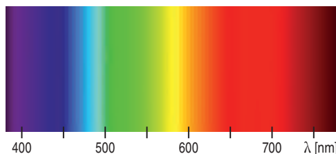
Obr. 1.4 Spektrální barvy a jejich vlnové délky, spojitě spektrum bílého světla
