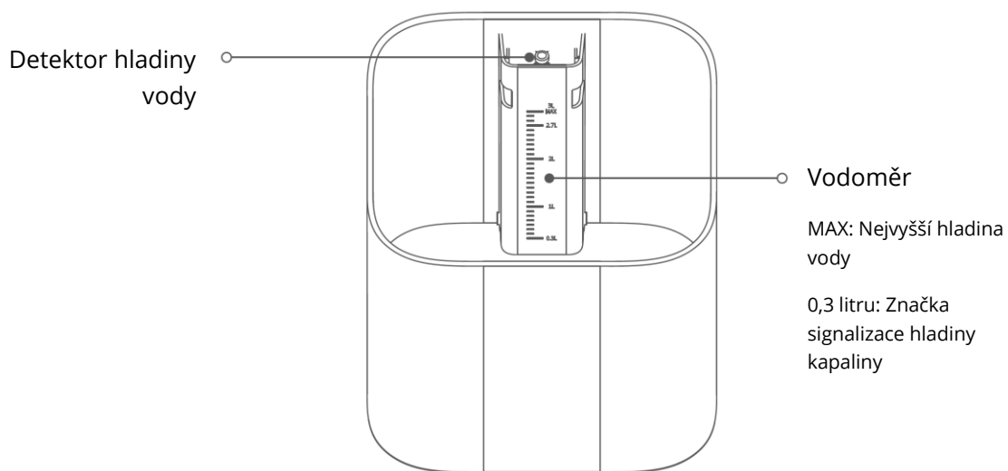
Sud na vodu
