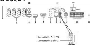
Obrázek 2-5 Připojení ovladače A
