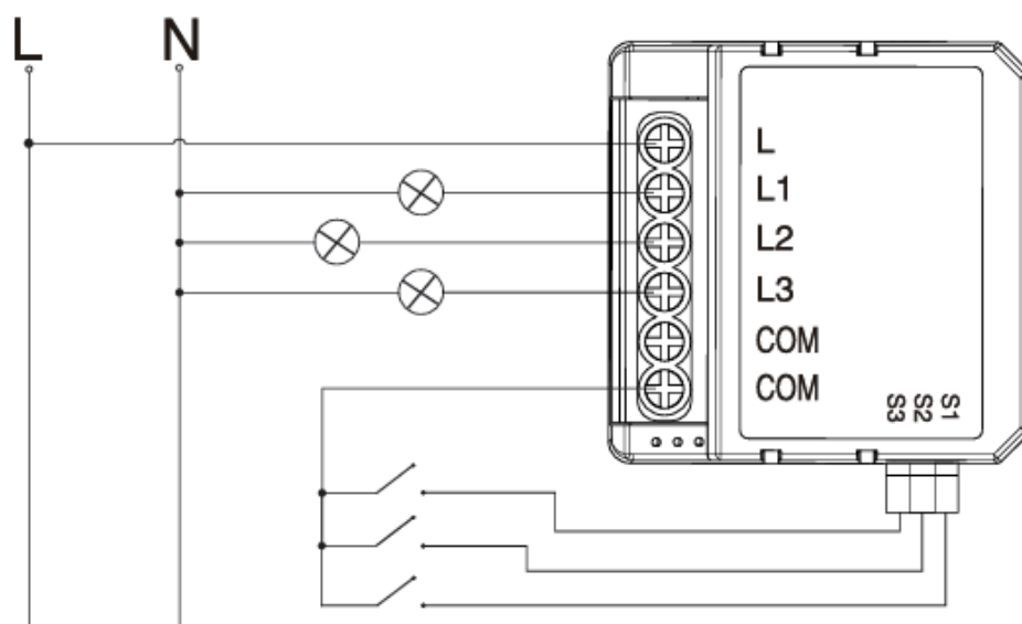
A szerelvények kapcsolási rajza (L1 L2 L3-ból az egyiket)
