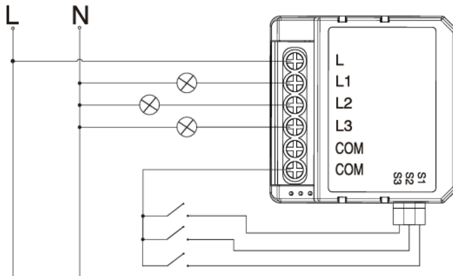
Verdrahtungsplan der Armaturen (L1 L2 L3 eine davon)
