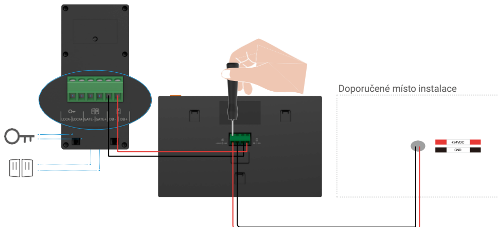
Schéma zapojení 1-1
