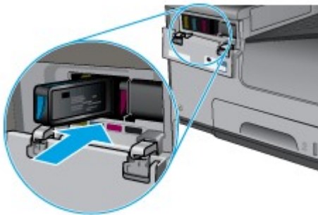
Abbildung 6: Einsetzen der Tintenpatrone
