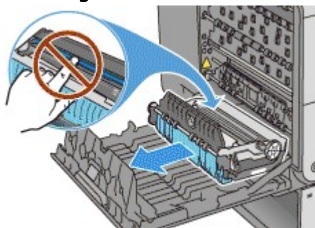
Abbildung 2: Entfernen der Tintenauffangeinheit
