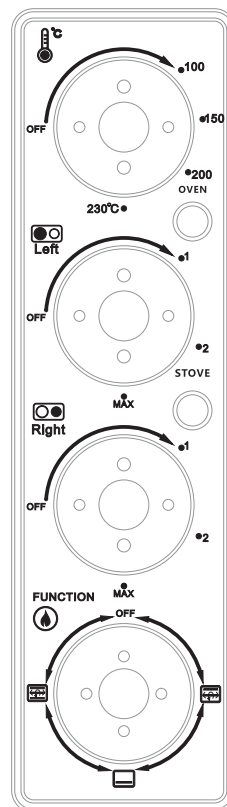
panel ovládání
