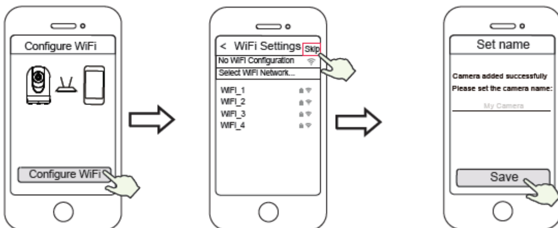
Wi-Fi konfigurálás
