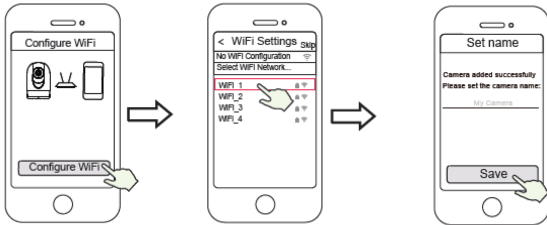
Wi-Fi konfigurálás
